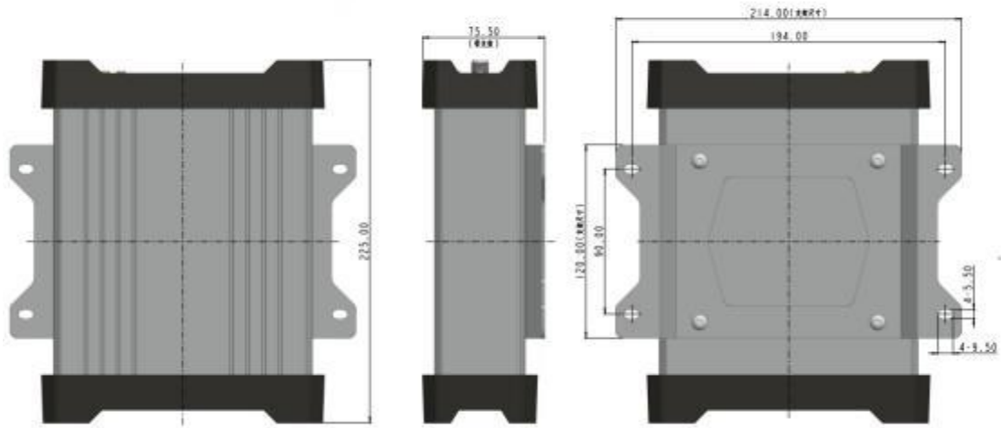
图 2-1 BDX-300Pro 外观尺寸
